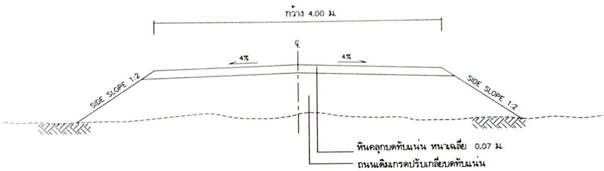
รูปตัดตามขวางงานลงหินคลุก
